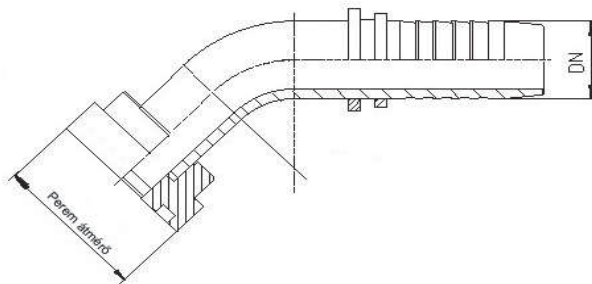
( CAT ) Armătură cu flanșă CATERPILLAR la 45°
